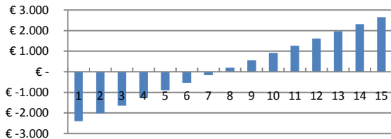
Grafiek terugverdiëntijd 7,2 jaar
